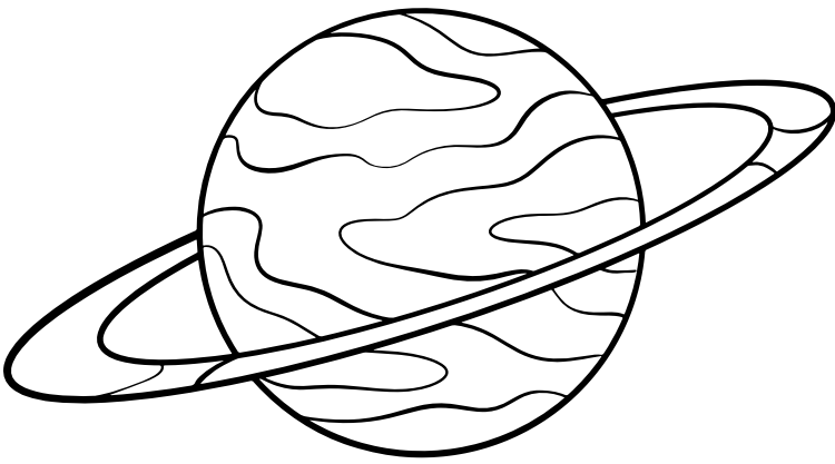
planet
